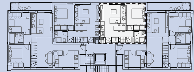
Planta tercera
