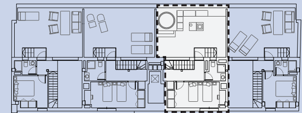
Planta cuarta
